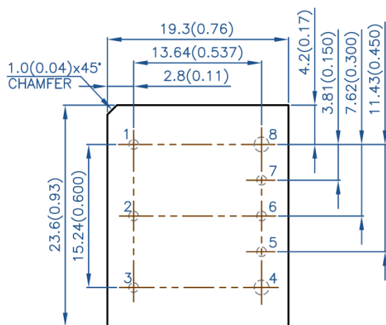
Open Frame Module
